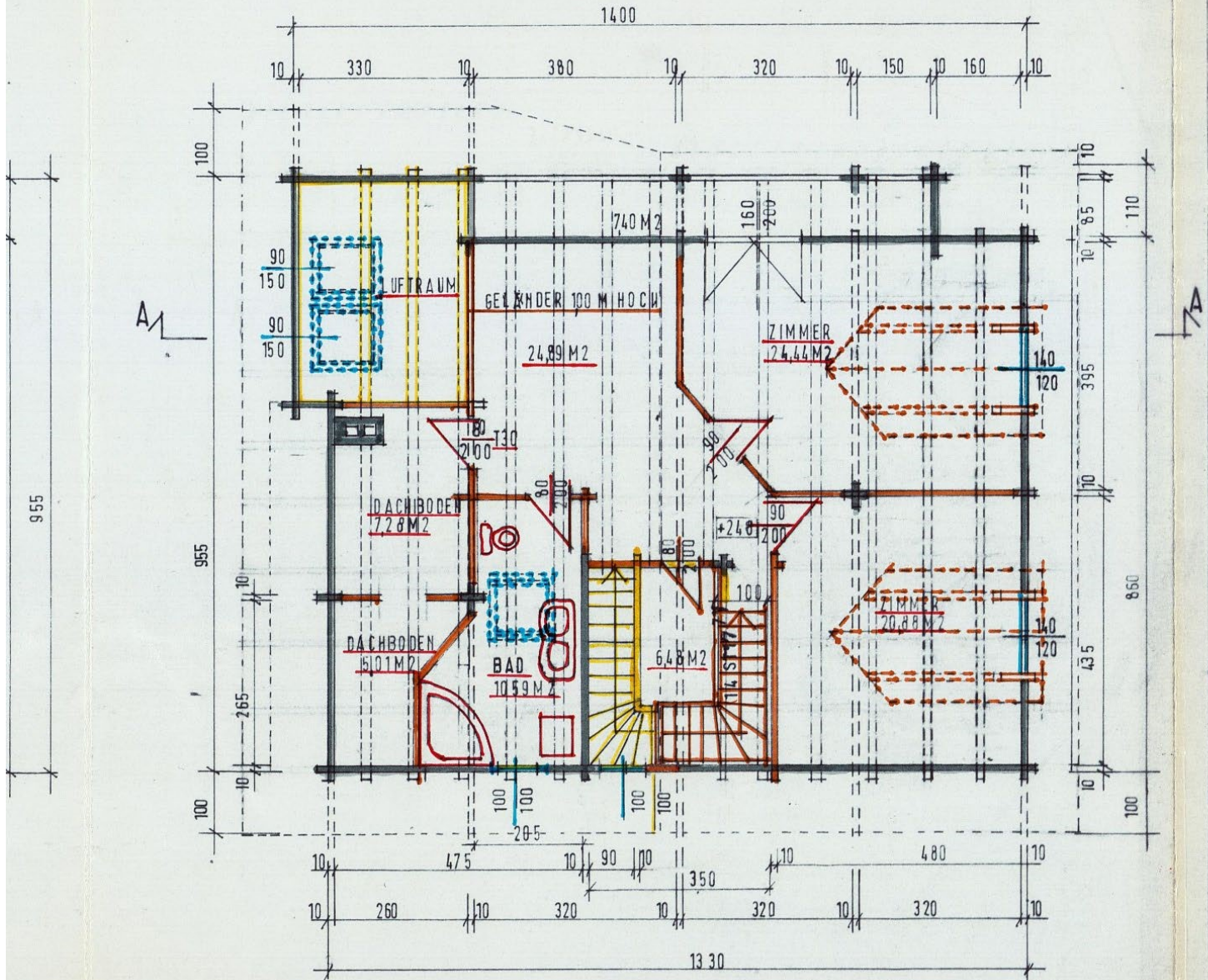
DACHBODEN DACHGESCHOSS
