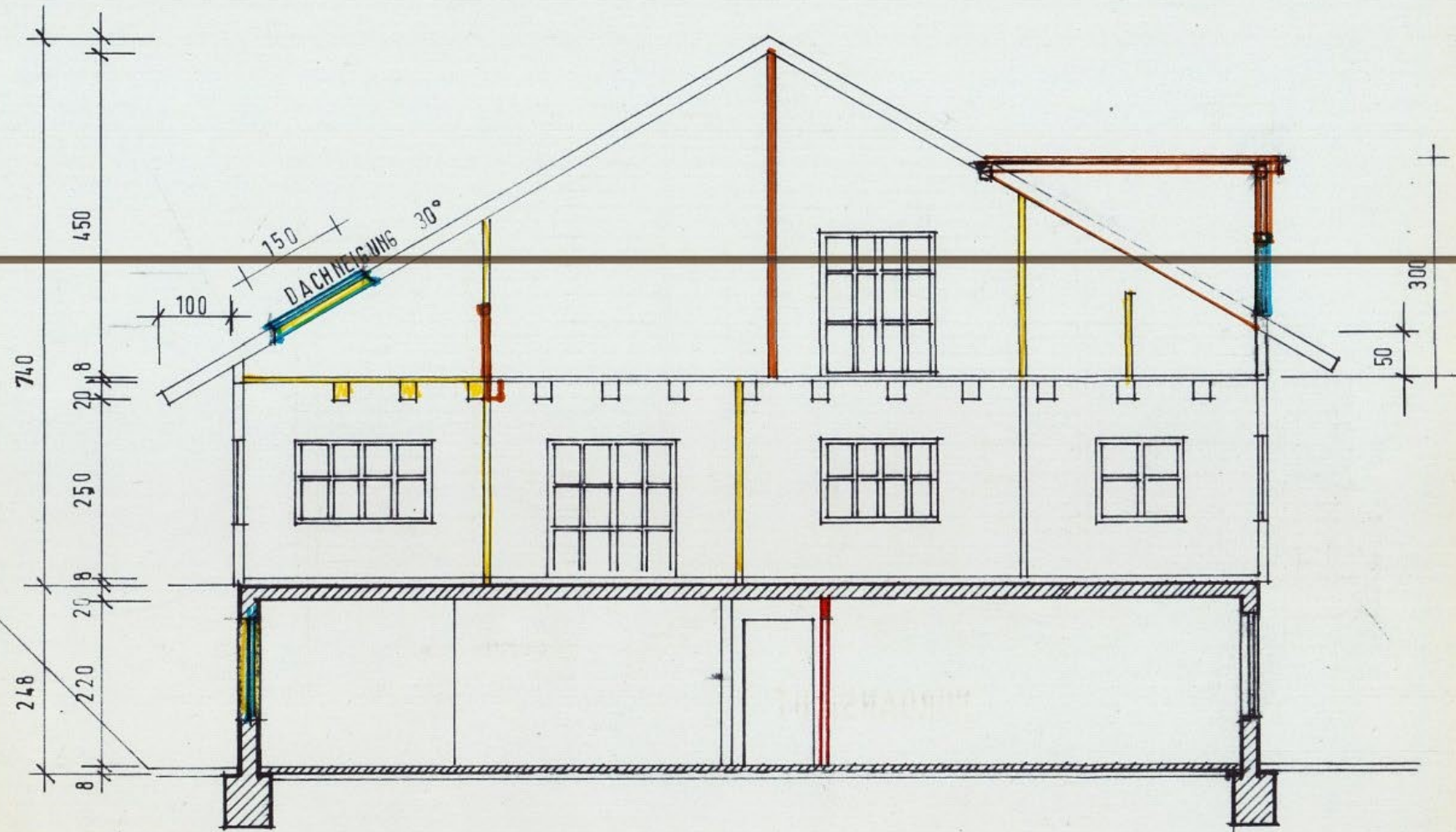
SCHNITT A-A
