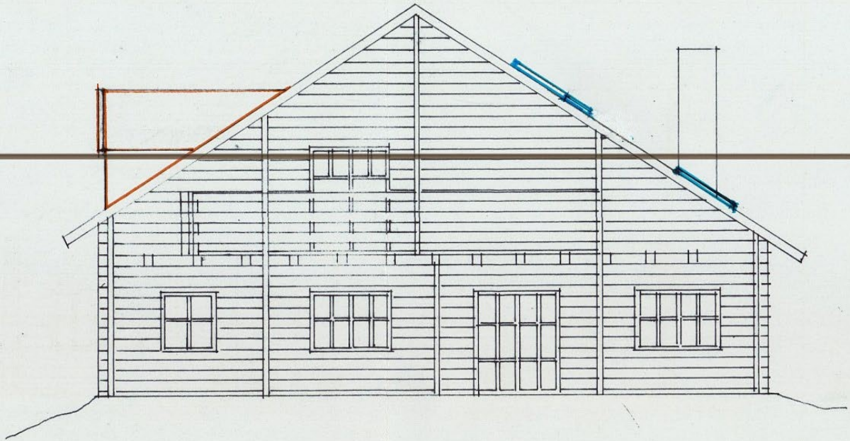
SÜDANSICHT
